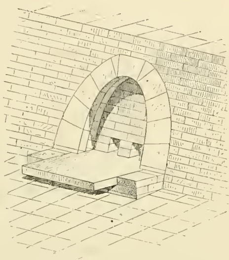
91. — Canal de Khorsabad à voûte elliptique, d'après le géométral de Place, t. III, pl. 39.
